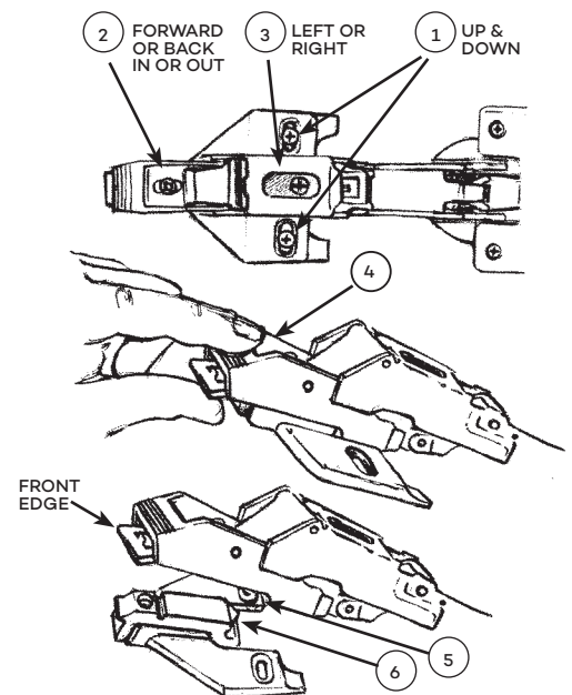
EASY-REACH HINGE
