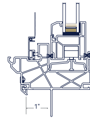
1" Mounting Fin Set-back
